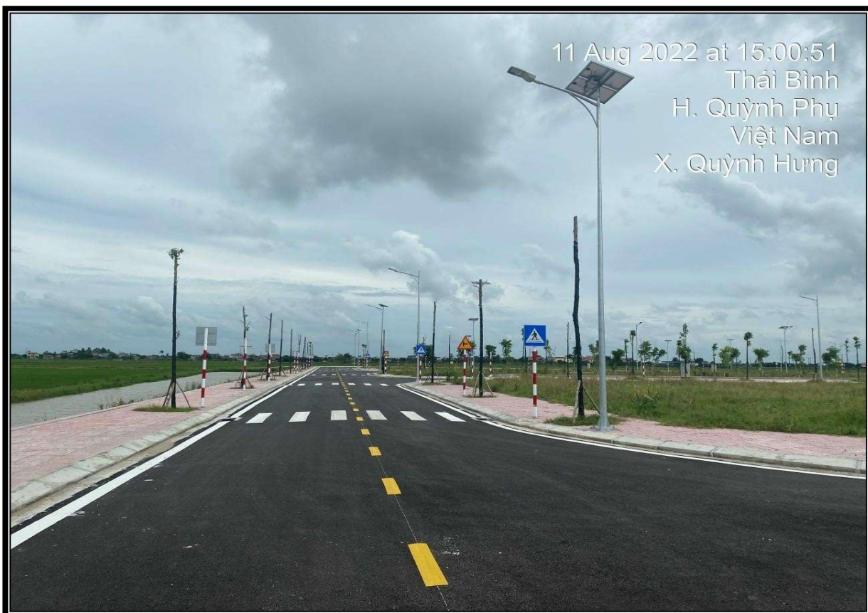
Đèn chiếu sáng năng lượng mặt trời tại Khu Dân Cư Quỳnh Hưng - X.Quỳnh Hưng – H.Quỳnh Phụ - T.Thái Bình
